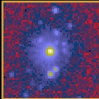
X-Ray : ROSAT
