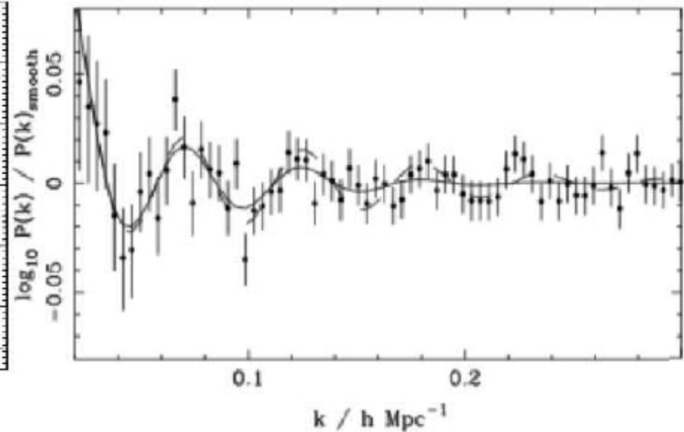
SDSS
